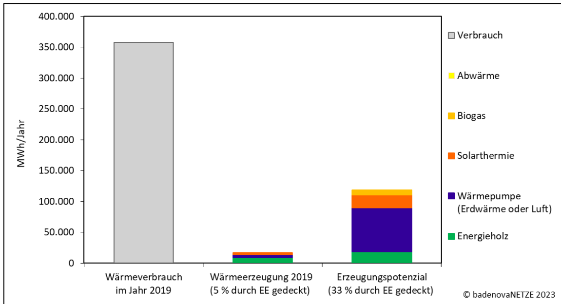
Abbildung 18 – Zusammenfassung erneuerbarer Wärmeerzeugung und Wärmepotenziale in Waldshut-Tiengen
